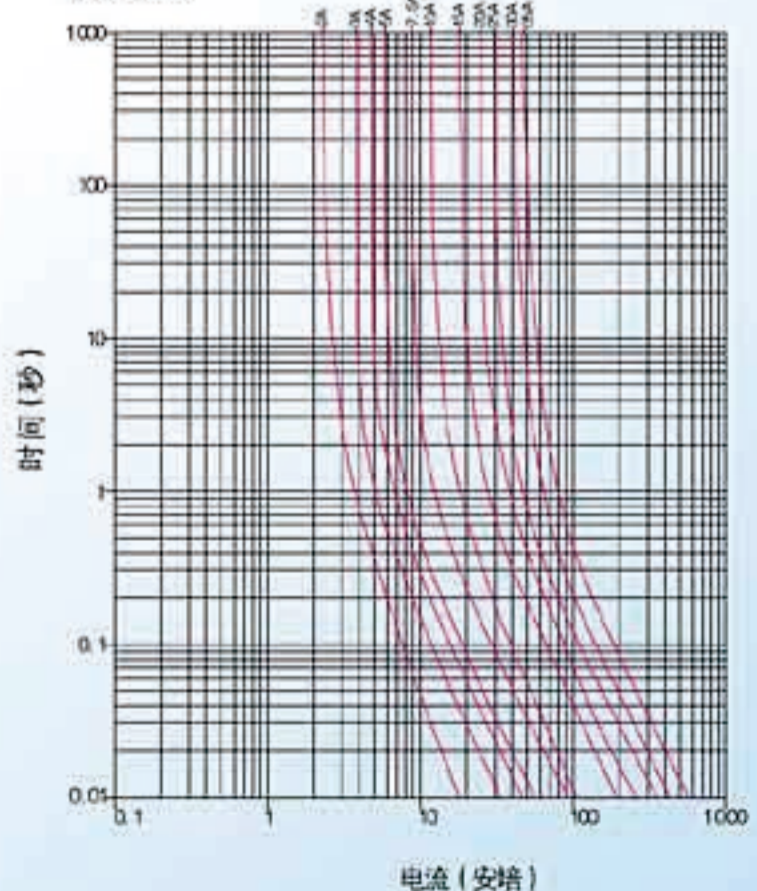
熔断特性
